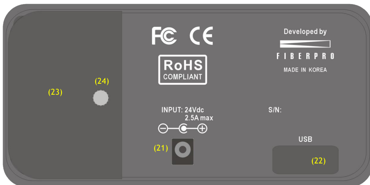
図 2: 背面パネル
