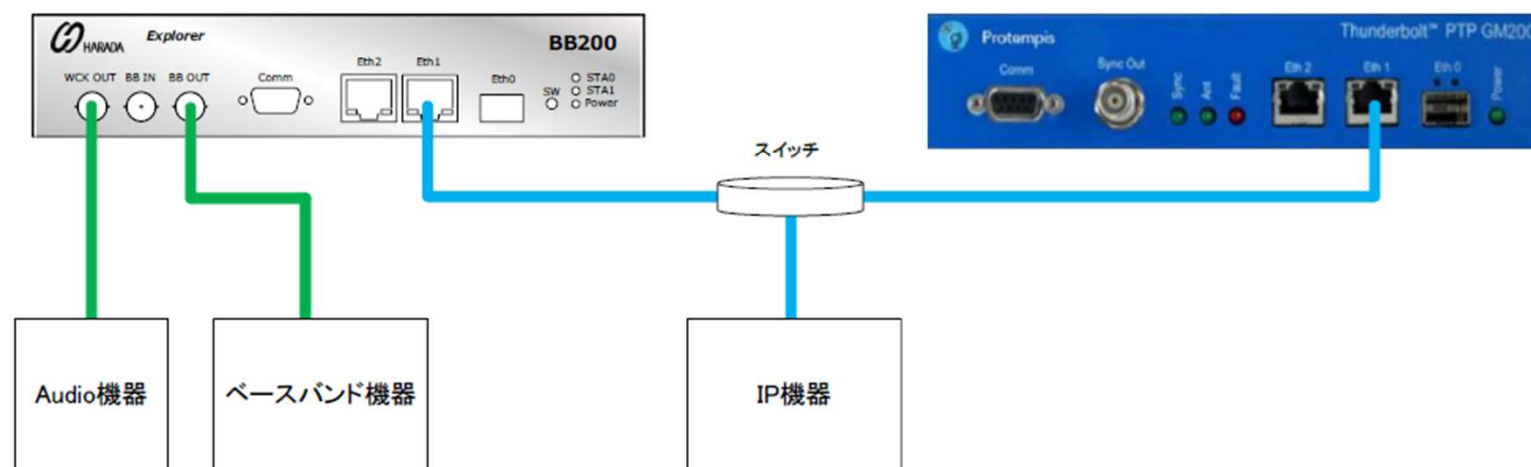
図 2 ローカルネットワーク接続
