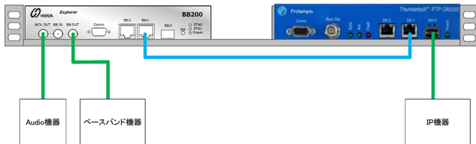
図 1 GM200MI としての接続例
